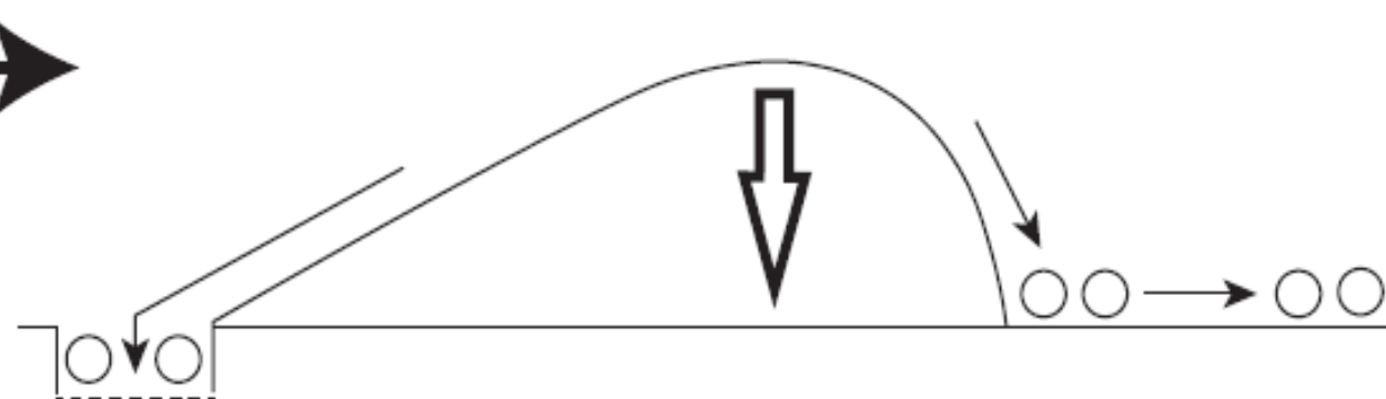
(d) Rainfall driven sediment redistribution
