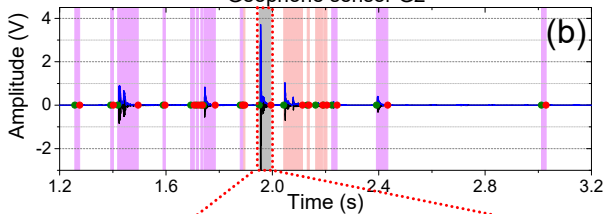
Geophone sensor G2
