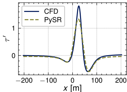
(d) Bump H/L = 0.4
