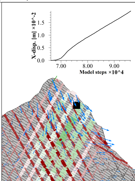
(d) \phi = 30^\circ , c = 0.05 MPa
