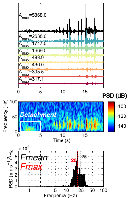
(d) Super-Sauze
