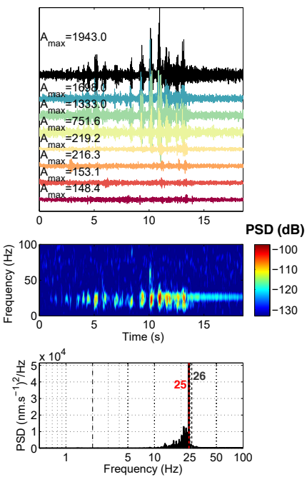
(d) Super-Sauze
