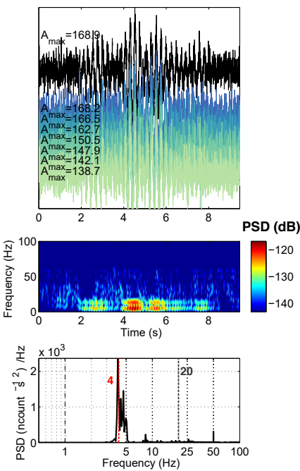
(d) Séchilienne
