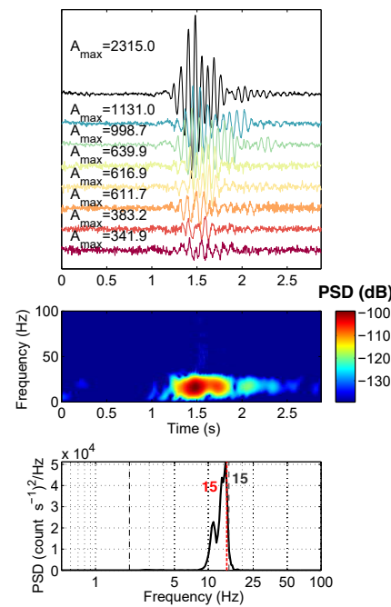
(f) Super-Sauze
