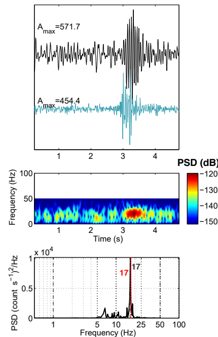
(f) Super-Sauze
