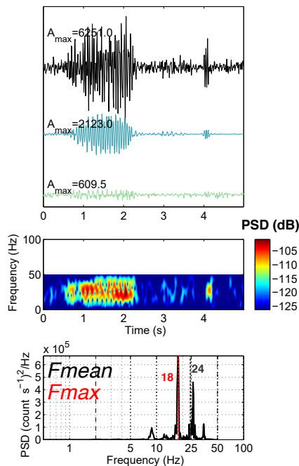
(d) Séchilienne
