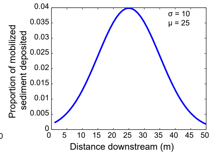
(d) Shortened Gaussian
