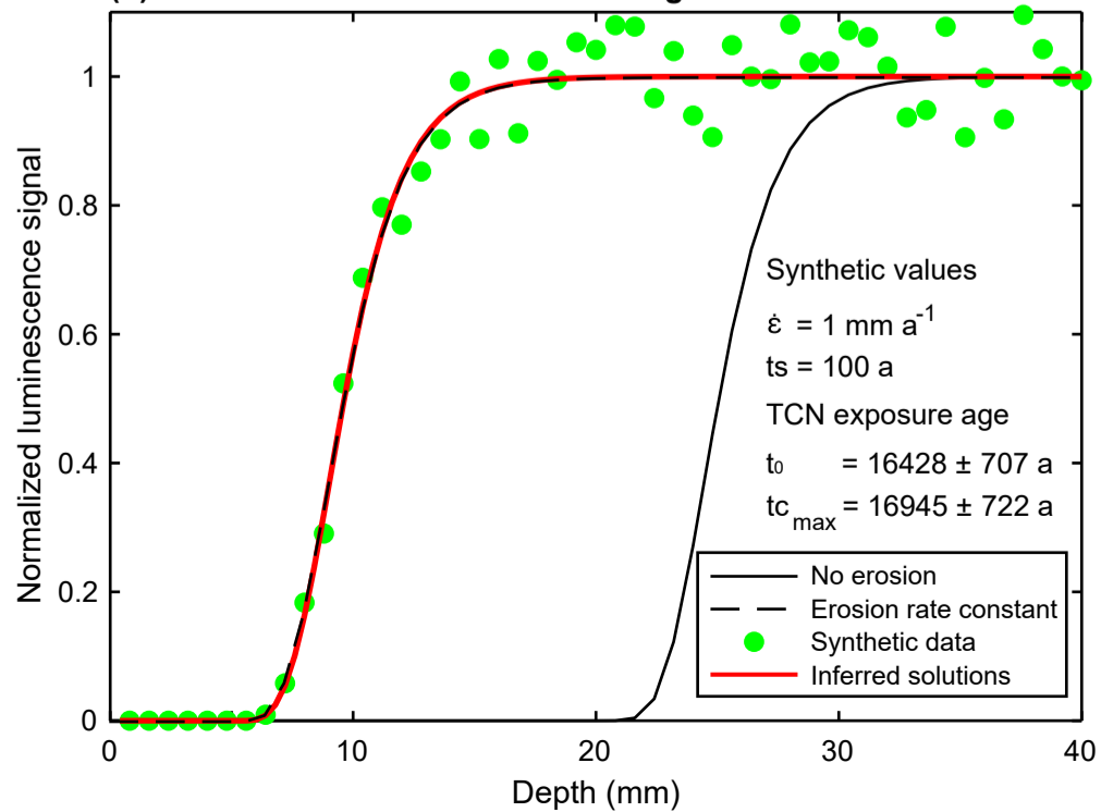
(d) Evolution of the luminescence signal
