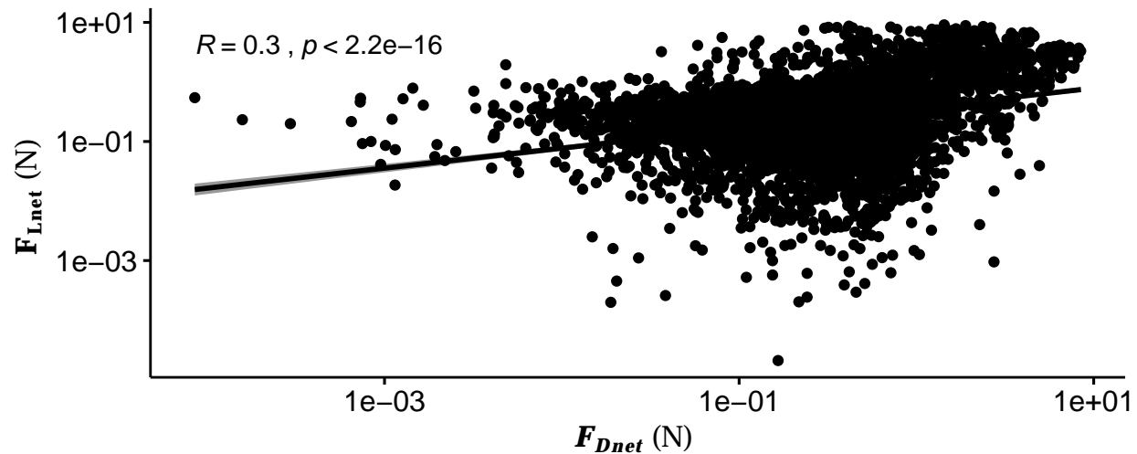
Ellipsoid (Lab)
