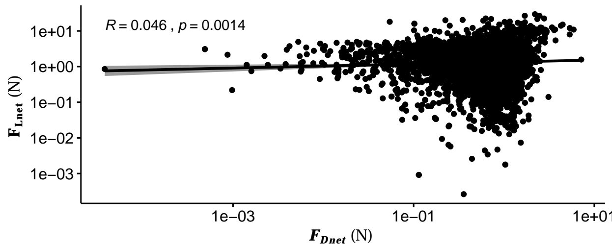
Ellipsoid (Erlenbach)
