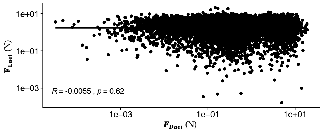
Ellipsoid (Erlenbach)
