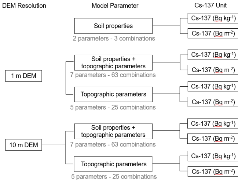
Fig. 9. GAM parameter combinations.
